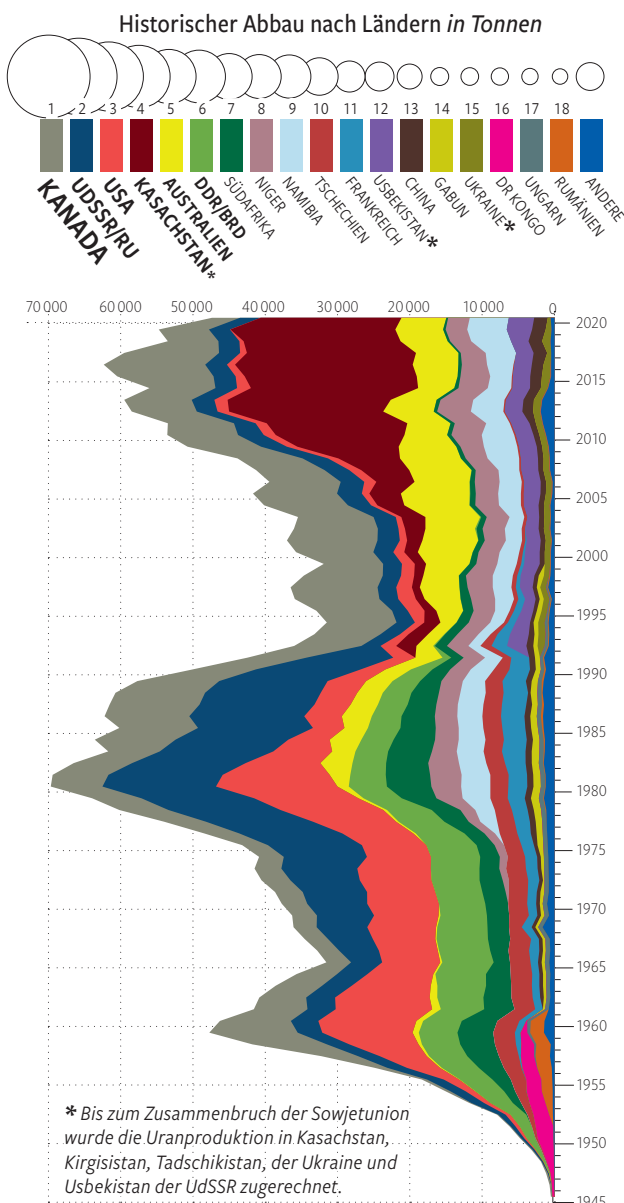
Uranproduktion 1945 bis 2020
